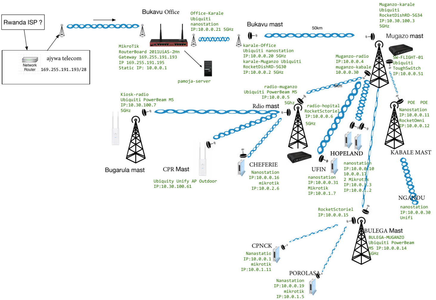
Figure 5 : Diagramme de réseau pour le réseau communautaire PamojaNet (Utilisé avec l'autorisation de La Différence)
