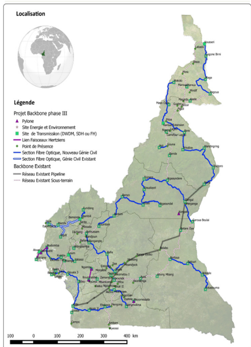
Figure 2 : Projet du backbone national en fibre optique phase III (CAMTEL 2019)
